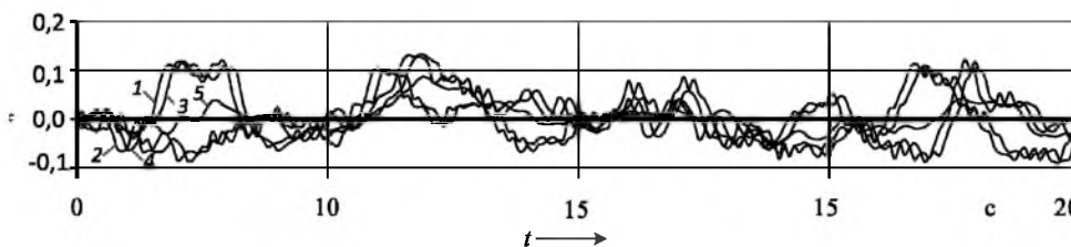
Рис. 5. Результаты моделирования вертикальной динамики автомобиля при движении его по дороге с микропрофилем со скоростью 20 м/с: 1 – z_1 ; 2 – z_2 ; 3 – z_3 ; 4 – z_4 ; 5 – z_c
